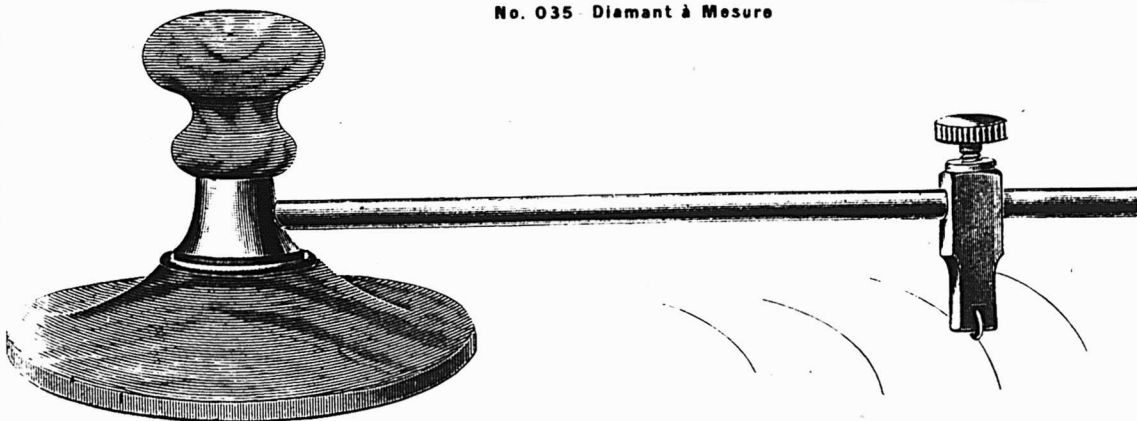
No. 6 - Diamant Circulaire, Coupe des Cercles de 3 à 20 pouces de diamètre
