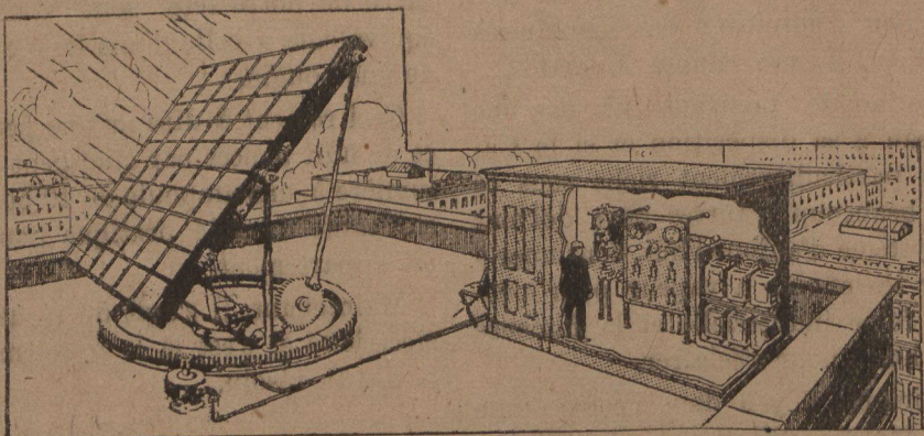
L'INSTALLATION COMPLÈTE. On voit à gauche, un récepteur formé de 60 cellules et supporté par un système d'orientation. A droite le logement des accumulateurs.
