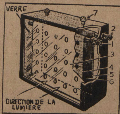
1 et 2, Bornes pour les fils. 3, Côté en verre. 4 et 5, Plaques de cuivre, 6, eau salée. 7, dégagement des gazs.
