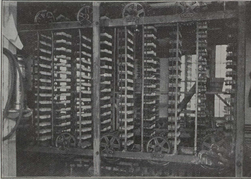
Dispositif mécanique, mobile, pour sécher les allumettes.
