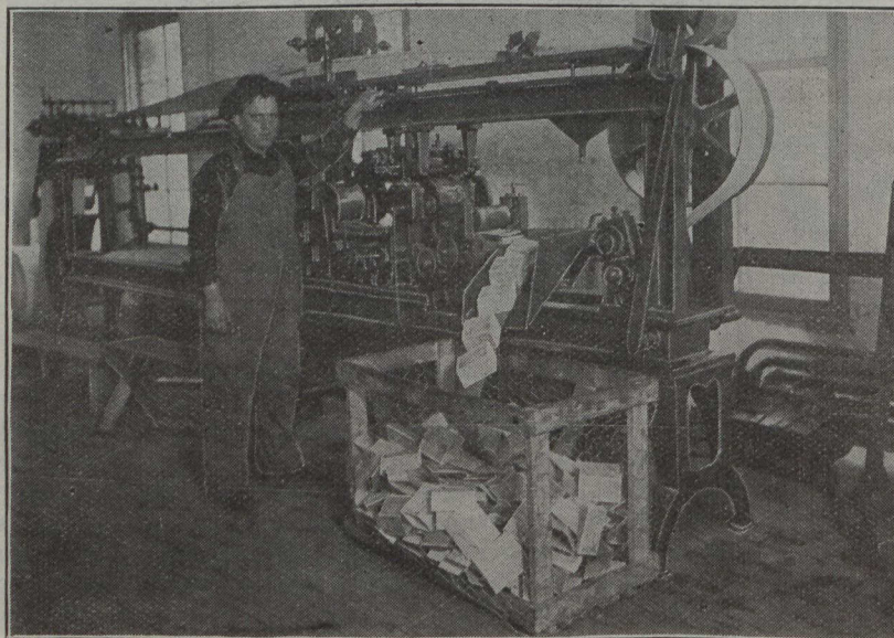
Machine à faire les boîtes d'allumettes. Cette machine fait la boîte, et imprime dessus ce qu'il faut pour en activer la vente.
