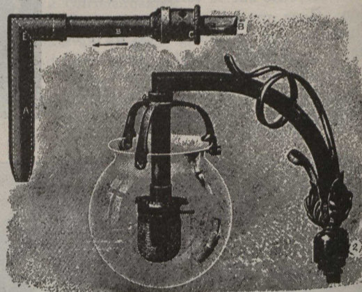
Bec à flamme renversée—1. Détails de construction. 2. Vue d'ensemble
