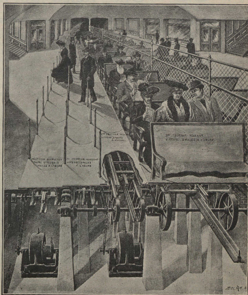
Vitesse de la plate-forme principale, pourvue de sièges, 9 milles à l'heure. Cette plate-forme, à elle seule, peut transporter 48,000 personnes, assises confortablement, par heure.
