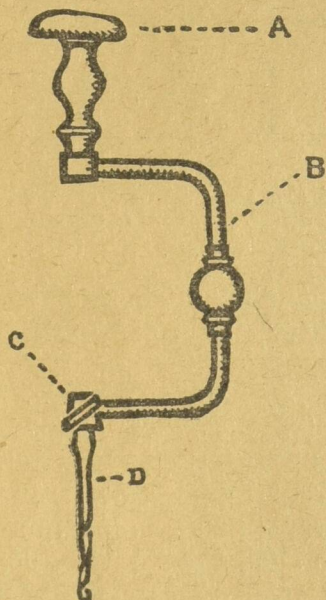
Vilebrequin où l'on voit en A la pomme, en B la soie, en C le fût avec sa vis de pression et en D la mèche fixée sur l'outil.
