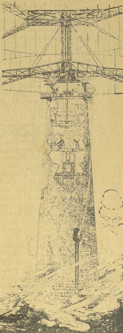
Profil du phare radiographique, montrant les ailes rotatives du sommet de la tour d'où partent les ondes. Les lettres du code sont émises par ces ailes, chaque point du compas ayant sa lettre correspondante.
