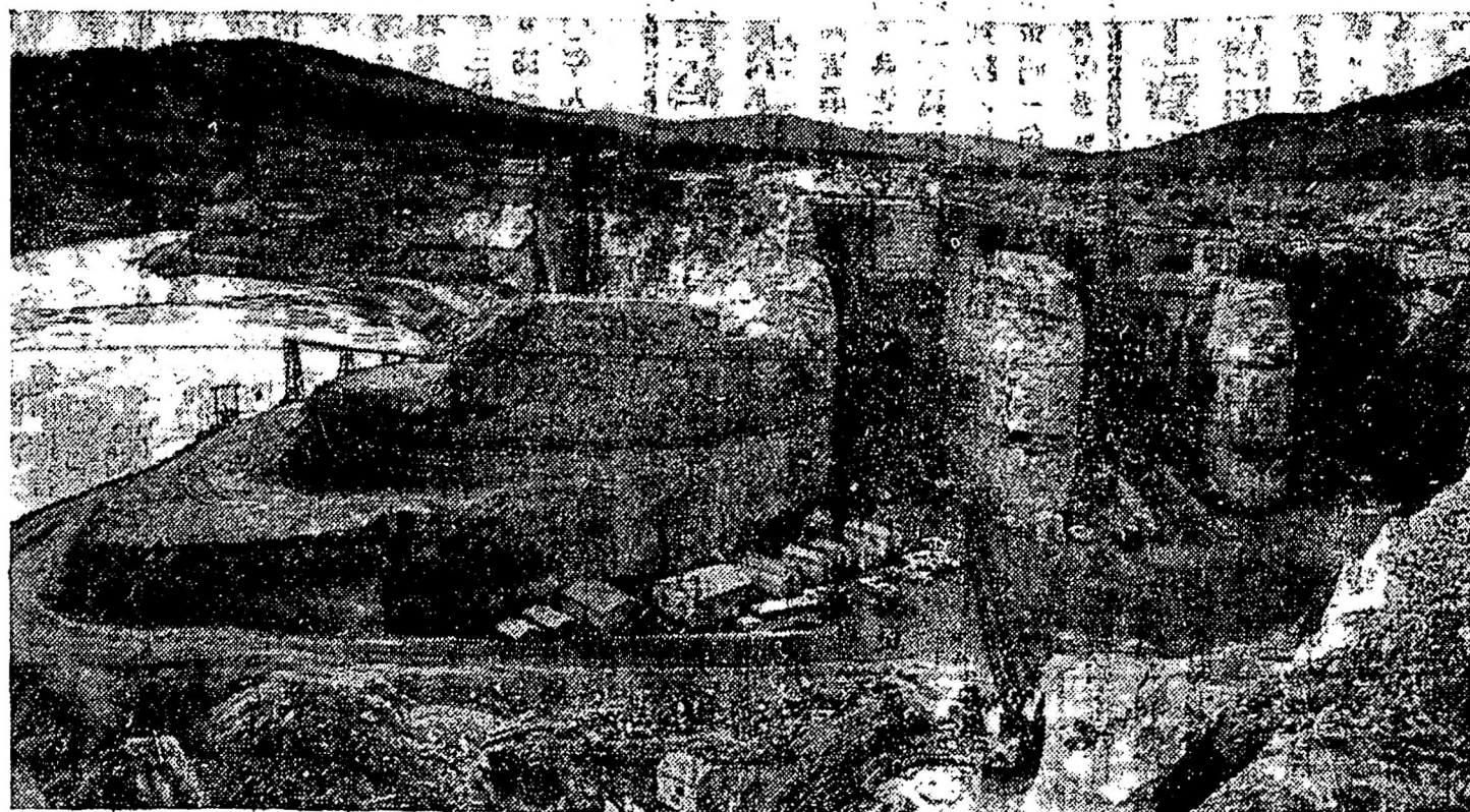
(附圖一) 在砵地治山區水閘工程中，那些巨大的改流隧道行將完成，數星期後，建築起六百尺高的水閘，偉大的和平河流域為之改觀。社會信託黨政府的兩河水力政策（指和平河與哥林比亞河同時發展計劃）將保證卑詩省成為北美洲最大的供應平價電力的寶庫。
