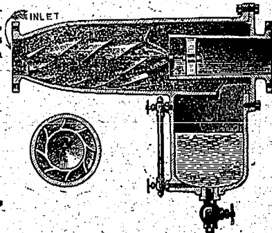
Horizontal Separator.
