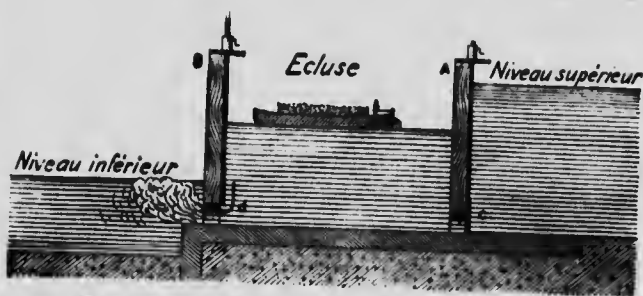
ECLUSE.—A et B, portes; C, vanne fermée; D, vanne ouverte.
