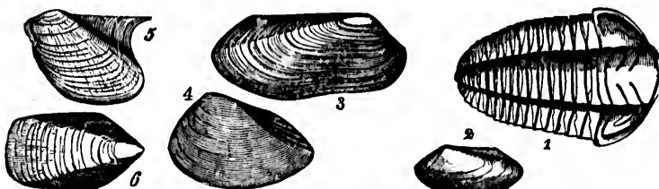
1, Calymene Beckii . 3, Orthonota ———. 5, Avicula ———.
