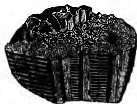
Columnaria alveolata , a fossil coral.
