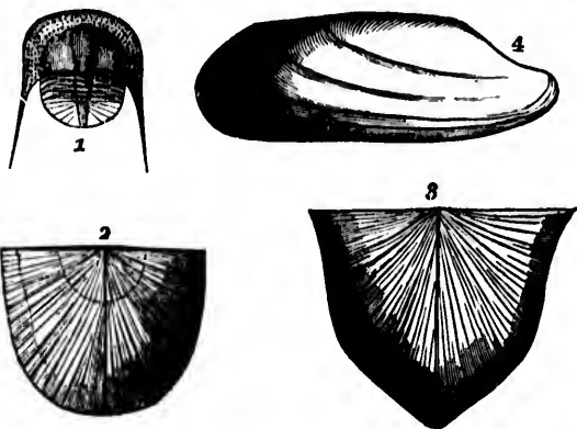
1, Trinucleus concentricus . 2, Leptaena deltoidea .
