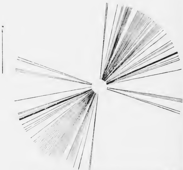
FIG. 9. Direction des veines de quartz montrées sur la carte des lots 10 et 11, concession II canton Tisdale dans la région Porcupine. L'orientation de la structure de la roche encaissante est représentée par la ligne noire
