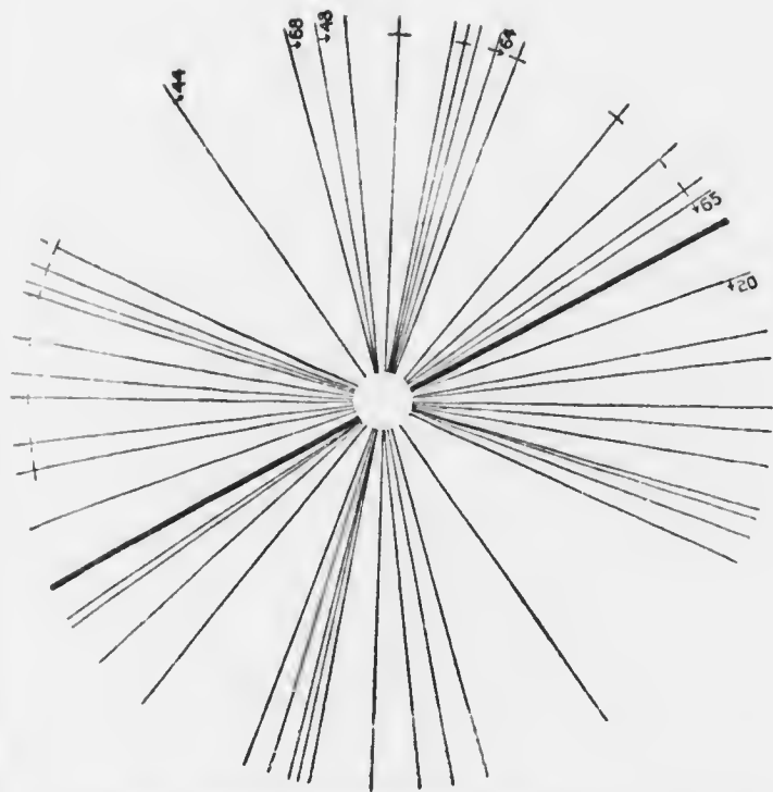
FIG. 8. Direction des veinules de quartz dans la dolomie ferrugineuse au nord du lac Larder, canton McGarry, district Nipissing Ontario. La direction structurale de la dolomie est indiquée par la ligne noire.
