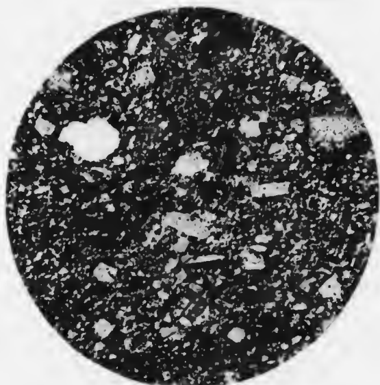
Photomicrographie de graywacke de la série Pontiac, du lac Clericy, Co de Pontiac, Qué. Nicols croisés. Grossissement 20 diamètres. A comparer avec les planches XVII et XVIII.
