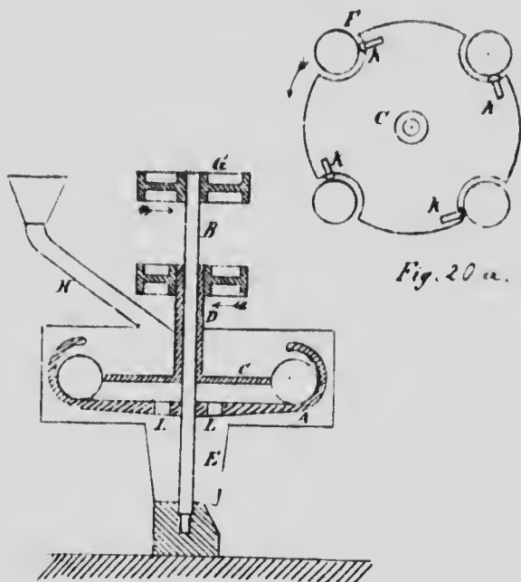
Fig. 20. Cannon Ball Mill.
