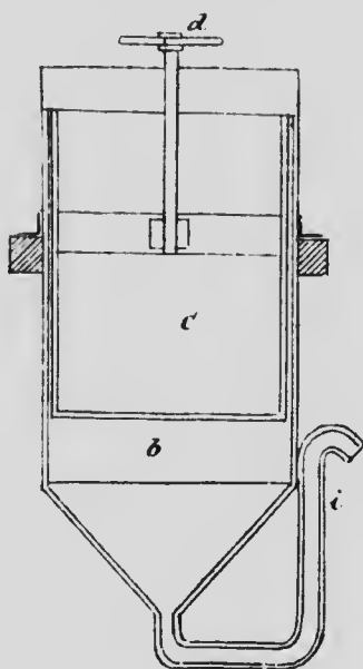
Fig. 29.—Spitzlütte.
