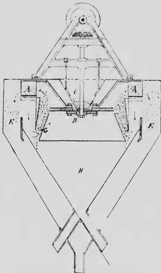
Fig. 26. Mumford & Moodies Separator.
