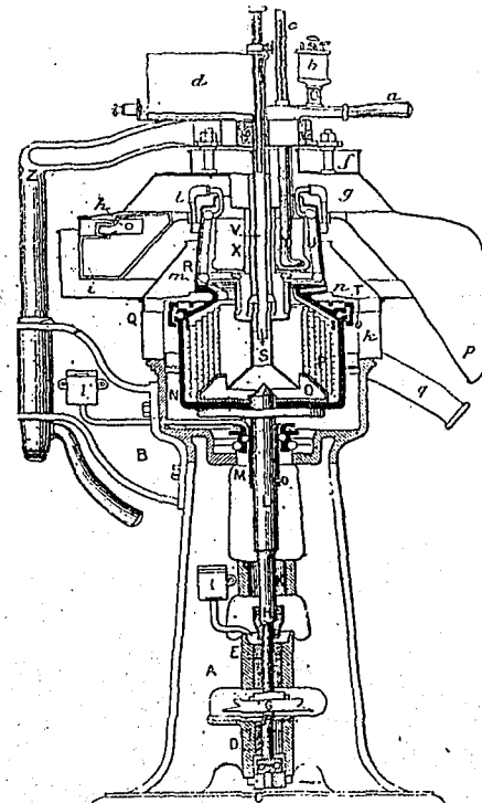
Coupe vertical du radiateur.—A, bâti; B, console du support à pivot; C, crapaudine à billes; D, coussinet inférieur de la commande; E, coussinet supérieur de la commande; F, arbre moteur; G, poulie de commande; H, tête de l'arbre moteur; I, graisseur; K, coussinet inférieur de l'arbre du bol; L, arbre du bol; M, coussinet supérieur de l'arbre du bol; N, bol d'écrémage; O, cône de distribution du lait gras; P, cadres réfrigérants du lait; Q, joint des deux chambres du bol; R, bol de barattage; S, arrivée du lait gras; T, arrivée de l'eau froide; U, cadres réfrigérants de la crème; V, conduit du lait gras; X, conduit de l'eau froide; Y, tube de barattage; Z, support à pivot; a, levier du tube de barattage; b, réservoir de matière colorante; c, thermomètre; d, réservoir d'alimentation du lait gras; e, tige du régulateur; f, réservoir d'arrivée de l'eau froide; g, chambre d'évacuation du beurre; h, racleuse d'évacuation du beurre; i, bassin de sortie de l'eau froide; k, bassin de sortie du lait écrémé; l, sortie de l'eau froide; m, conduit de la crème; n, conduit du lait écrémé; o, joint étanche; p, sortie du beurre; q, sortie du lait écrémé.
