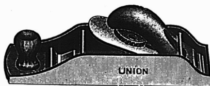
Rabot debout "UNION" No 137. Ce Rabot, tel qu'indiqué dans la gravure ci-dessus, est réversible; il est pourvu de deux lumières et de deux assises par la lame. No 137, longueur 8 pouces, lame 1 1/2 pouces.
