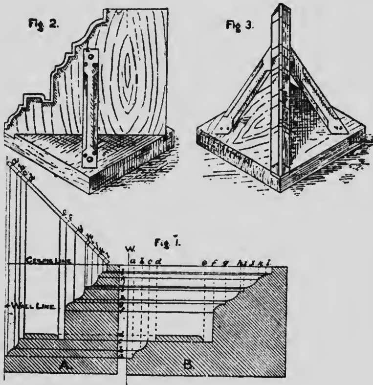
-MITRE-MOULD.
