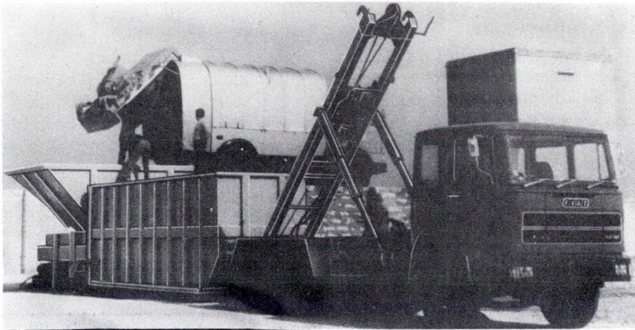
Sistema de transferencia de residuos sólidos de la firma Atlas Hoist and Body.
