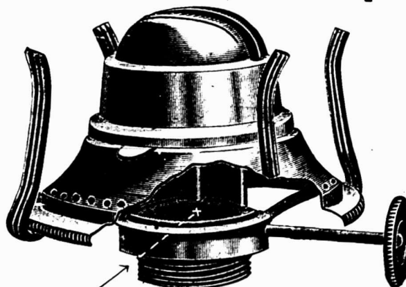
Brûleur Banner pour Kérosène.
