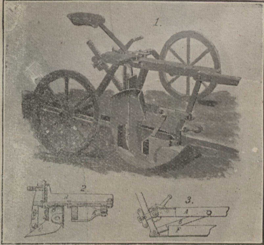
Une machine à creuser des fossés
