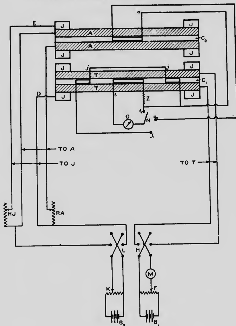
Fig. 6. Connexions pour essais de perméabilité.
