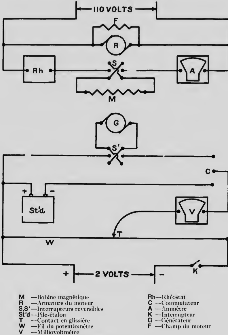
Fig. 3. Diagramme des connexions.
