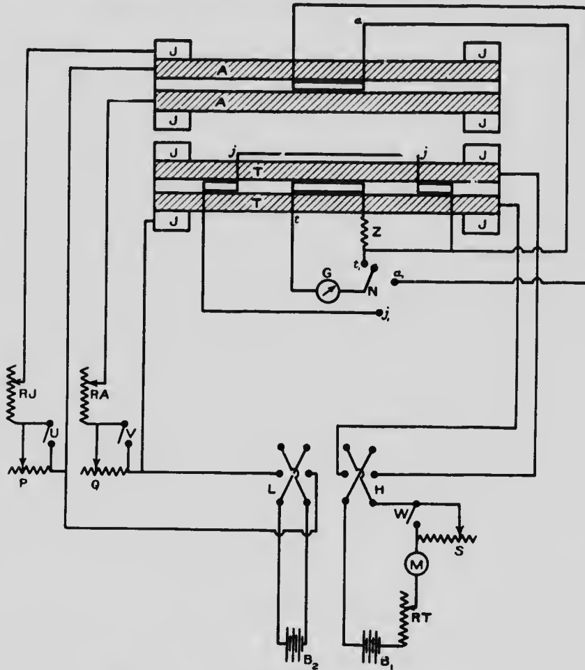
Fig. 7. Connexions pour expériences d'hystérésis.
