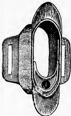
FIG. 422.—Tube of Dieterichs; posterior view.
