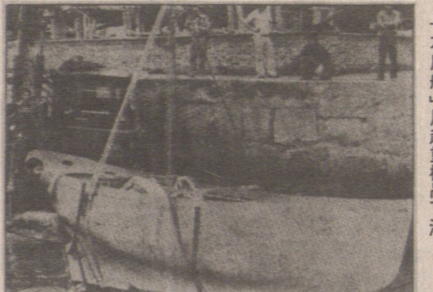
「石屎船」用起重機吊下海
