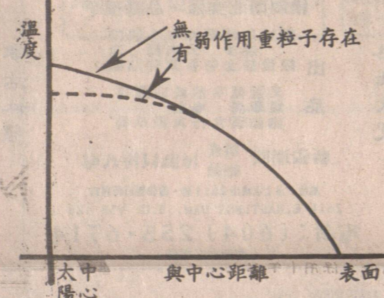
太陽中心與中心距離與溫度。
