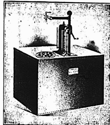
GRAVURE No. 9—Outillage de Premier Plancher pour Huiles non Lubrifiantes.
