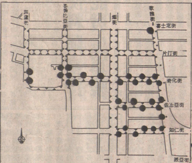
美化華埠街燈計劃簡圖
