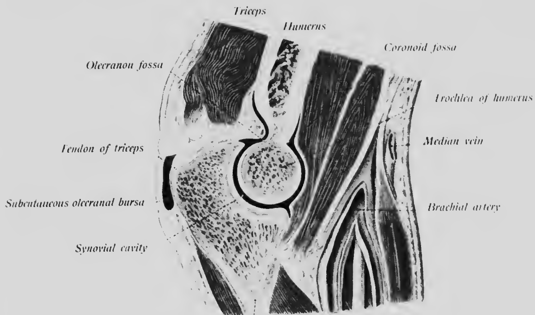
Ulna Fig. 201.
