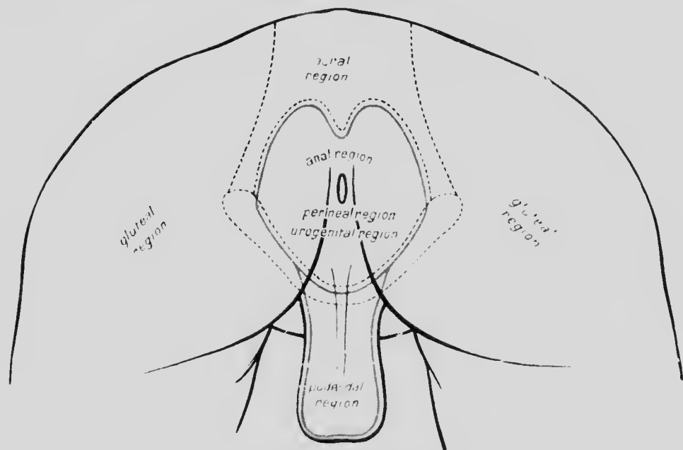
Fig. 234. Male perineum.
