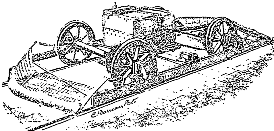
FIG. 1.—Train d'une voiture avec son moteur, la caisse enlevée, indiquant le bati glissant sur le rail et auquel est attachée la navette qui fait le contact dans le canal souterrain.
