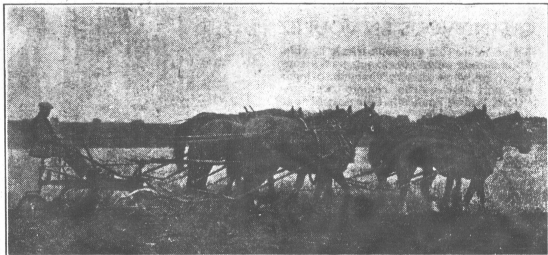
Sur la ferme, l'emploi de machines à plus forte capacité de rendement se vulgarise assez vite. Ainsi la charrue à une oreille se voit remplacée par les charrues sulky à deux, trois et même quatre versoirs. On voit ici sur une de nos bonnes fermes canadiennes une charrue à deux sillons. (Courtoisie de Massey-Harris & Co. Limited).
