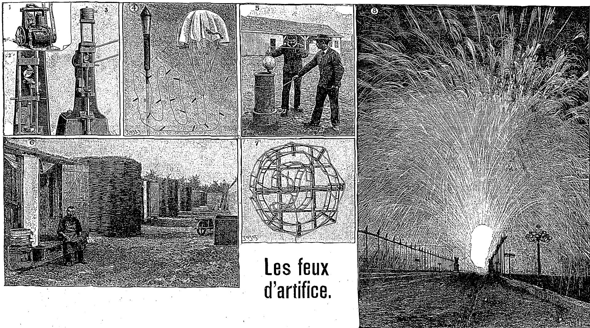
Fig. 1—No. 1 Machine à comprimer les étoiles. Fig. 2 et 3—Machine à charger les fusées et détail du mécanisme. Fig. 4—Fusée à parachute. A—Parachute plié. B—Baguette. E—Fusée. Fig. 5—La bombe d'artifice. Fig. 6—Baraques d'isolement pour la fabrication des feux d'artifice. Fig. 7—Pièce d'artifice décorative formée de lances. Fig. 8—Un bouquet de dix mille fusées.
