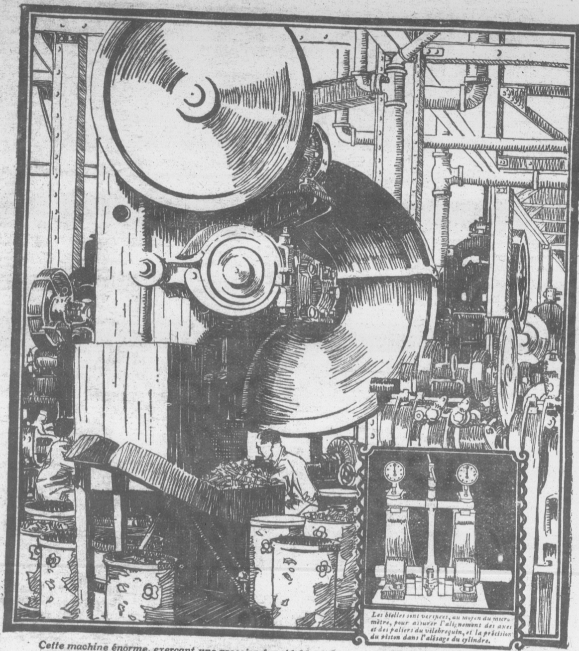
Cette machine énorme, exerçant une pression formidable, force chaque bielle à être forgée d'une forme et d'une épaisseur appropriées, comme préliminaire à 26 autres opérations mécaniques d'affinage.
