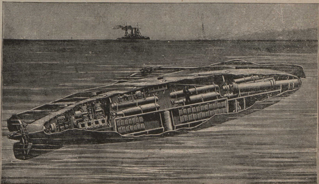
Le sous-marin "Fulton" acheté dernièrement aux États-Unis par la Russie. Ce navire vient, en manœuvrant, d'être avarié à Cronstadt. Notre gravure montre longitudinalement les appareils et machines, tels qu'ils sont à bord du "Fulton" en cours de route libre.
