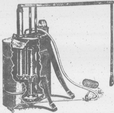
Pulvérisateur havresac, se portant sur le dos; le bras de pompe passe au-dessus de l'épaule de l'opérateur.
