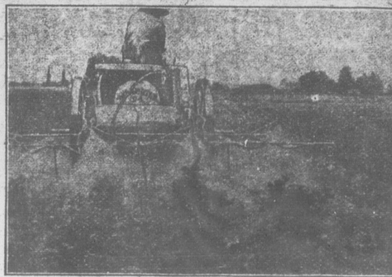
Pulvérisateur sur wagon à 4 roues arrosant 4 rangs. Les uns sont mus par les roues, les autres par un moteur.
