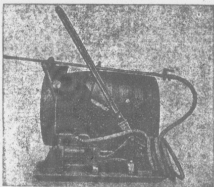
Pompe montée sur baril (vertical ou horizontal); se transporte sur voiture ordinaire. On peut ajouter tubulure pour 4 rangs, ou un bambou pour l'arrosage des arbres.
