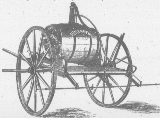
Pulvérisateur sur wagon à deux roues avec tubulure pour arroser quatre rangs à la fois. Celui-ci a une pompe à main; il s'en trouve avec pompe mue par un engrenage sur les roues.
