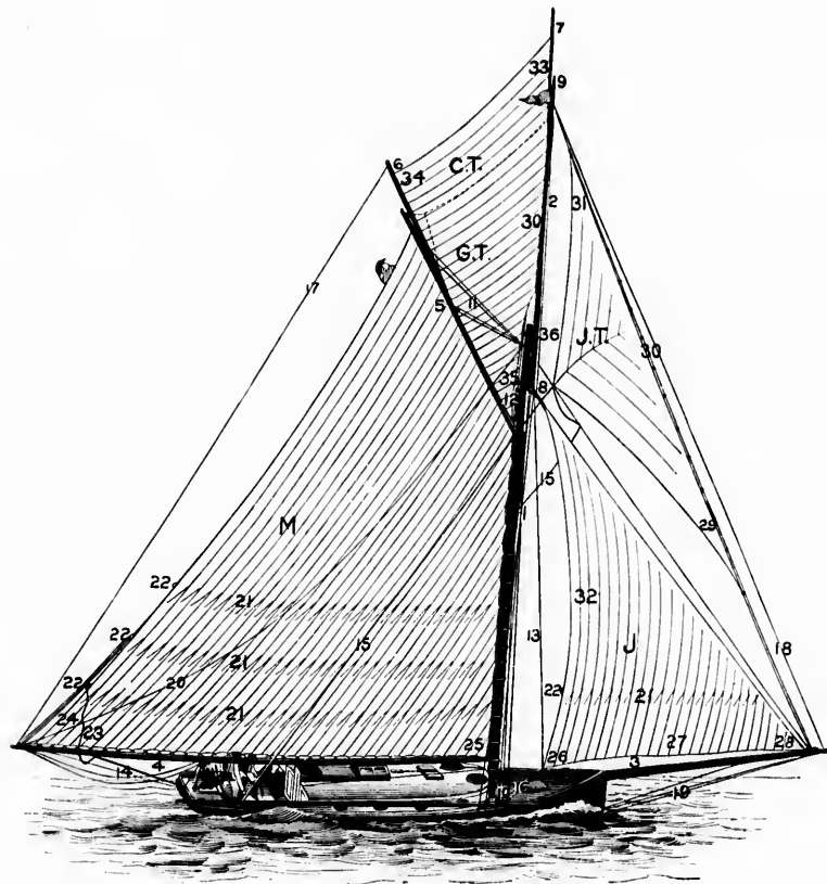
SLOOP YACHT.—FIGURE 100.
