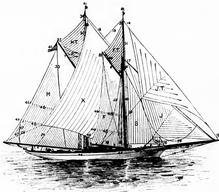
SCHOONER YACHT.—FIGURE 192.
