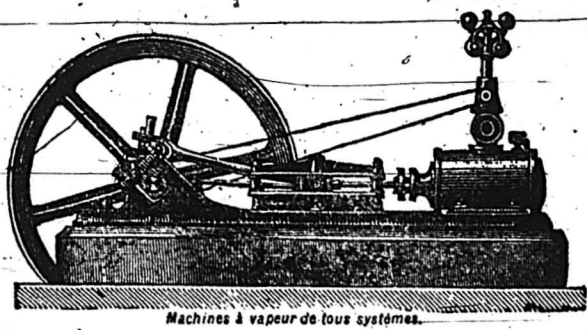
Machines à vapeur de tous systèmes.
