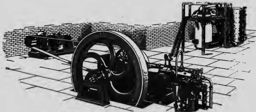
Fig 8.—Moteur Crossley de 200 chevaux avec gazogène, actionnant une dynamo.
