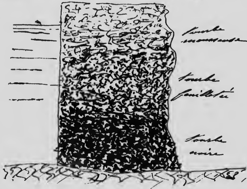
Fig. 1.—Coupe verticale d'une tourbière.
