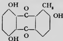
Emodin.
