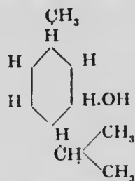
Menthol.
