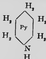
Piperidine.
