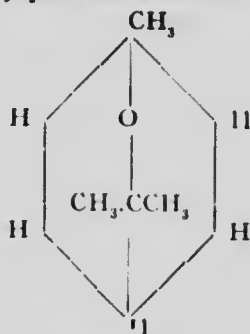
Eucalyptol.
