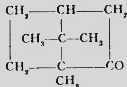
Camphor.
