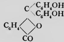
Phenolphthalein. Purgen.
