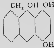
Chrysarobin.
