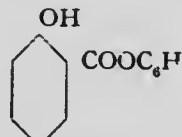
Salol.
