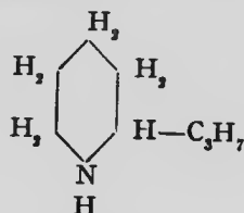
Coniine.
