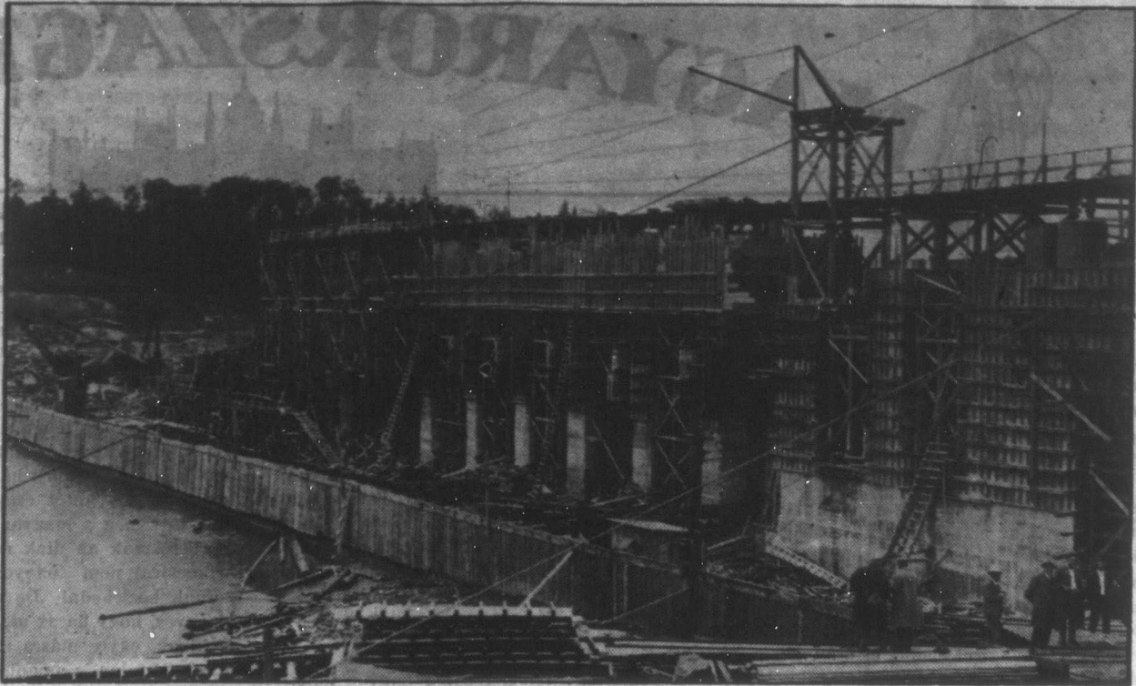
A Winnipeg Hydro Pointe du Bois mellett épülő 530 láb hosszú, vasbetonból készült villamos áramfejlesztő telepének alapjait mutatja képünk. A százezer lóerőnél is többejtő turbógenerátorok 132 ezer voltos áramot termelnek, melyet a szükséghez képest letranszformálva fognak szállítani, nemcsak Winnipegre, de a környező farmokra is. Jelenleg több mint 600 — köztük sok magyar honfitársunk — is dolgozik a telepen és észre legalábbis 800 munkásnak tud a Hydro megépítését nyújtani. Emellett olcsó villamos árammal fogja ellátni egész Manitoba déli részét s az ipar áram árának leszállításával is csökkenteni fogja a munkanélküliséget. A Winnipeg Tribune szívesességéből.
