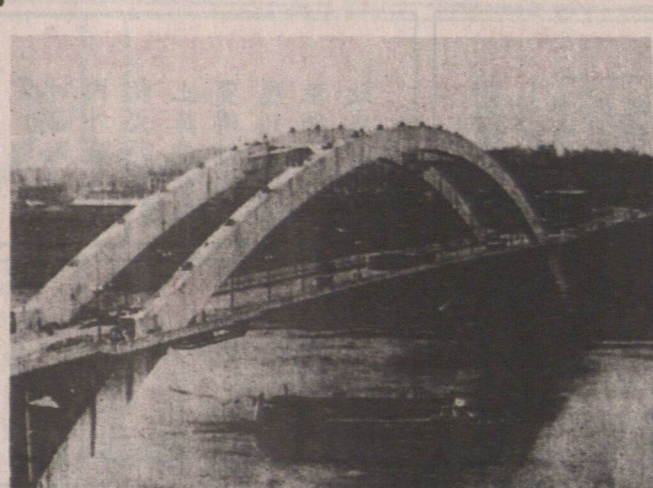
最大拱橋 目前世界最大跨徑二百四十米的中承式鋼筋混凝土拱橋，在四川省宜賓長江上建成，於七月一日通車。 (中新社傳真 趙永桂攝)
