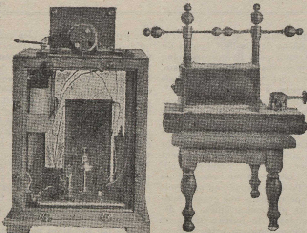
Ensemble des pièces servant à la distribution du courant électrique.
