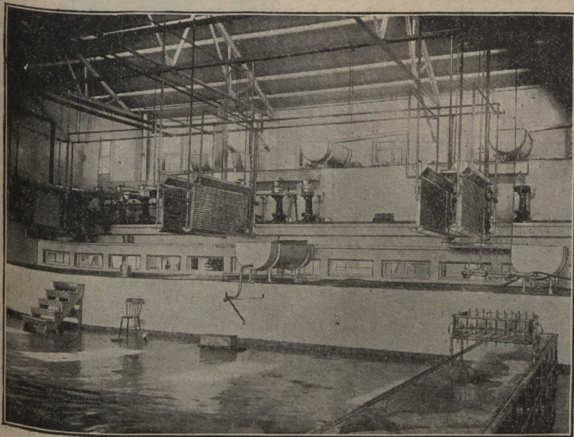
Réfrigérateur coulisse pour le lait et la crème. Au fond les séparateurs, à droite l'embouteilleur
