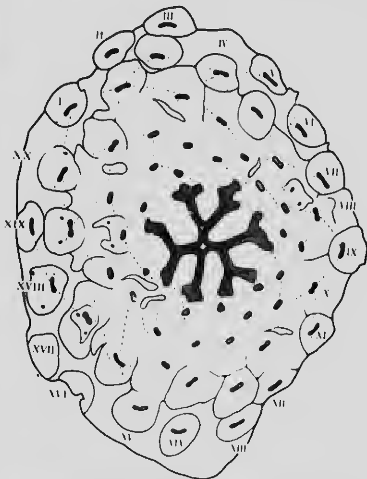
FIG. 2.— Asterochloa lura , var. Solmsi , P. Bertrand.—Section transversale du stipe montrant la disposition verticillée des traces foliaires. Les lignes pointillées représentent les hélices foliaires. Les nombres de I à XX désignent les séries radiales de traces foliaires.
