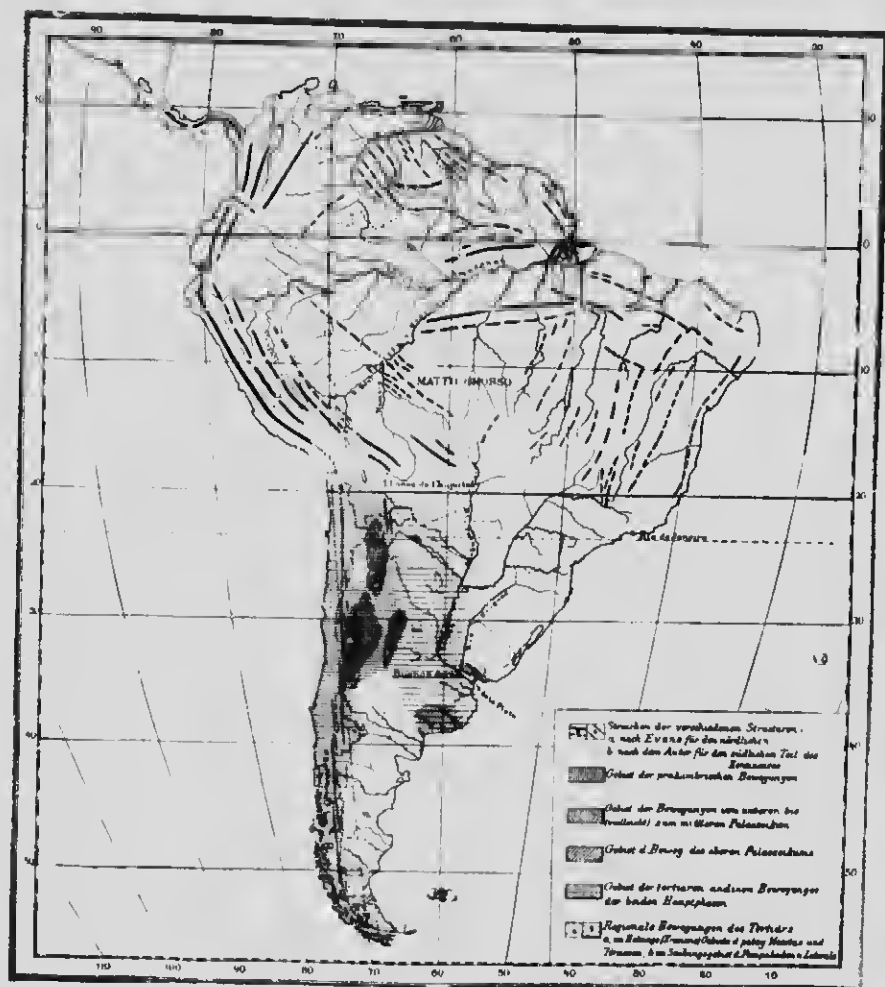
FIG. 1.—Tektonische Kartenskizze des südamerikanischen Kontinentes
