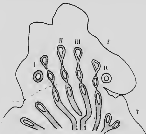
FIG. 4.— Chadoxylon radiatum , Unger, sp. — Fragments de tige montrant l'émission d'une trace foliaire. (D'après la préparation No. 15871 du Jernya Street Museum de Londres).
