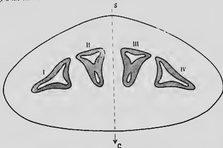
FIG. 5.— Cladoxylon dubium , Unger.—Section transversale d'un pétiole primaire coupé près de sa base, montrant la structure de la trace foliaire.
