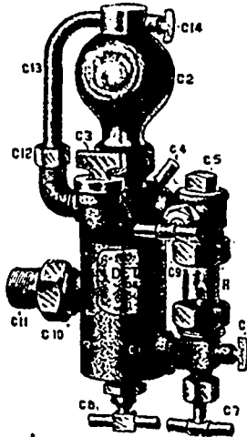
ZERO LUBRICATOR.
