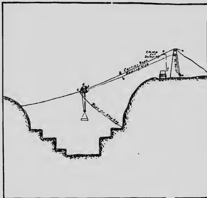
(Fig. 11.)—Mode d'exploitation d'un gisement d'amiante d'après Cirkel.
