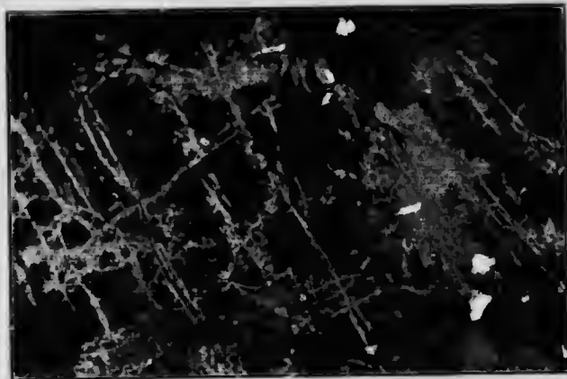
(Fig. 8.)—Veines d'amiante dans la roche.
