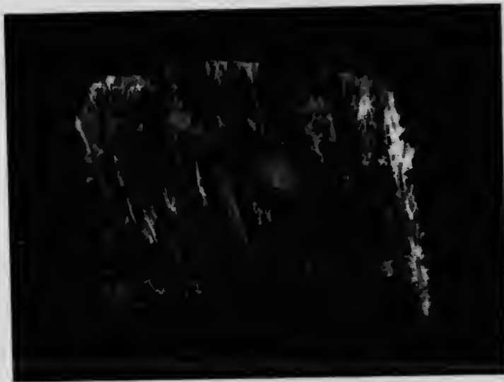
(Fig. 5.)—Amiante Chrysotile du Canada.
