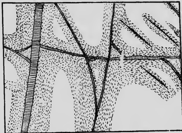
(Fig. 7.)—Mode de formation des veines d'amiante.
