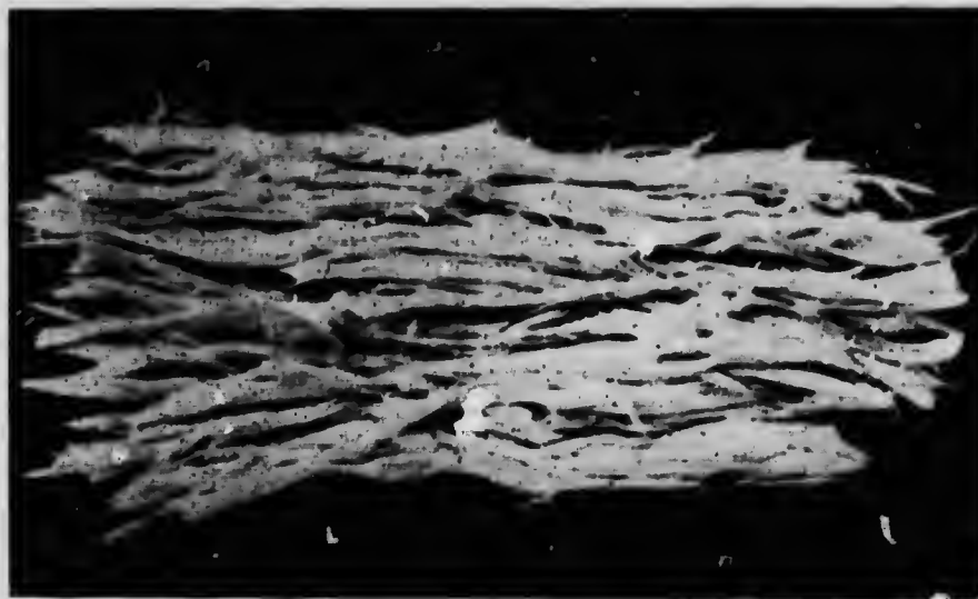
(Fig. 2.)—Amiante italien.
