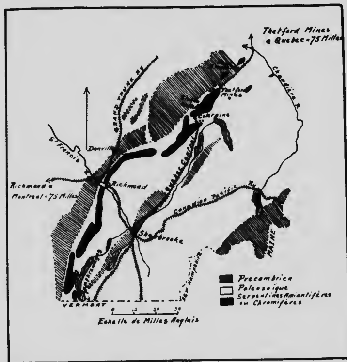
(Fig. 6.)—Carte-croquis de la région amiantifère de la Province de Québec d'après Dresser.
