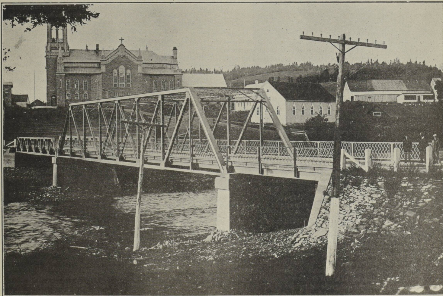
PAYSAGE ET SCÈNE DU TERROIR. — Pont sur la rivière Causapsal, à Causapsal, Matapédia. Ce pont à superstructure métallique et tablier en béton armé a une longueur totale de 245 pieds, formée de trois travées, la travée centrale ayant 130 pieds et les deux autres 70 pieds et 30 pieds respectivement. La largeur de la voie charretière est de 18 pieds, avec un trottoir de 4 pieds et 6 pouces en amont. Ce pont a été érigé en 1926.
