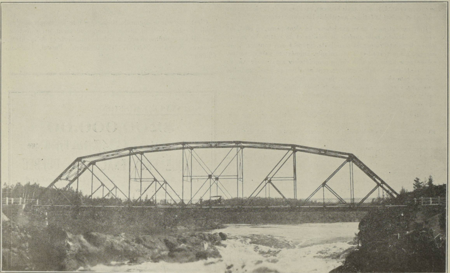
PAYSAGE ET SCÈNE DU TERROIR. — Pont au-dessus des chutes de la Grande Rivière Péribonca, à Ste-Monique (Honfleur), comté Lac S.-Jean. Pont à superstructure métallique de 200 pieds de longueur et de 18 pieds de voie charretière libre. Le tablier est en béton armé. Pont érigé en 1925.
