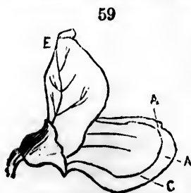
Fig. 59. Corolle papilionacée (Pois), E, étendard; A, A, ailes; C, carène.
