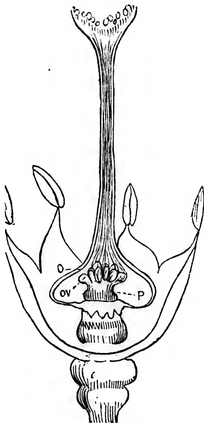
Fig. 83. Pistil du Celosia argentea très grossi, pour montrer les phénomènes de la fécondation. Les grains de pollen tombés sur le stigmate, envoient leur tube pollénique suivant toute la longueur du canal styloïde, pour arriver dans la cavité de l'ovaire o ; arrivés là, les tubes polléniques se mettent en rapport avec les ovules ov , que supporte le placentaire p .
