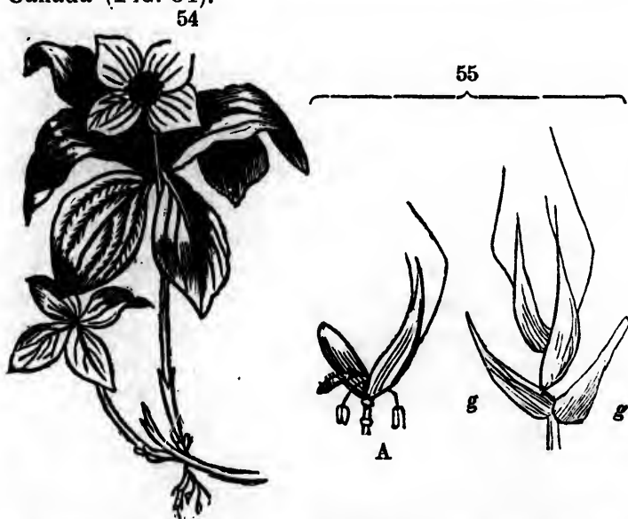
Fig. 54. Involucre simulant des pétales (Cornouiller du Canada).
