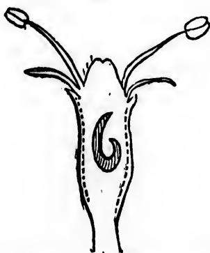
Fig. 61. Insertion hypogyne des étamines (Ancolie).
