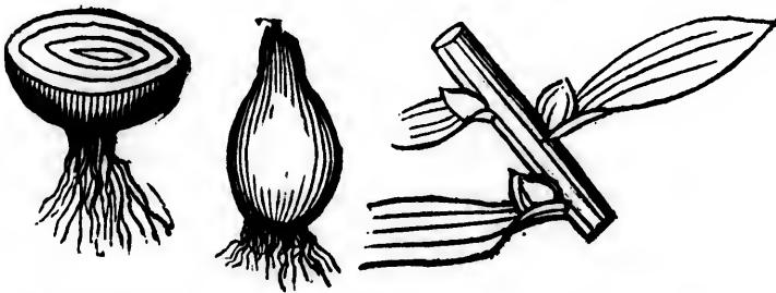
Fig. 31. Rhizome souterrain (Sceau de Salomon).
