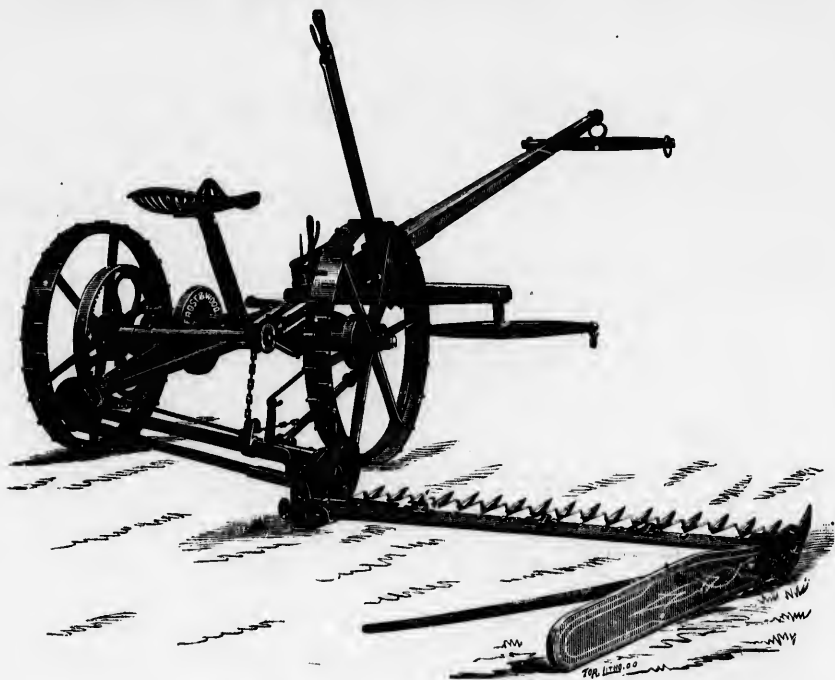
Faucheuse à faux en arrière Frost &amp; Wood
