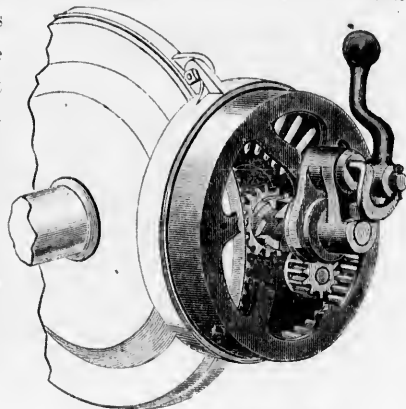
Changeur d'engrenage.
