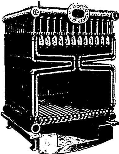
NO. 43. 1890 - U. S. PATENT NO. 434,227.
