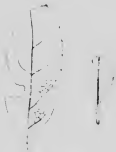
FIG. 20. Rhamnus quilchenensis n. sp. Leaves from Quilchena. x VI.
