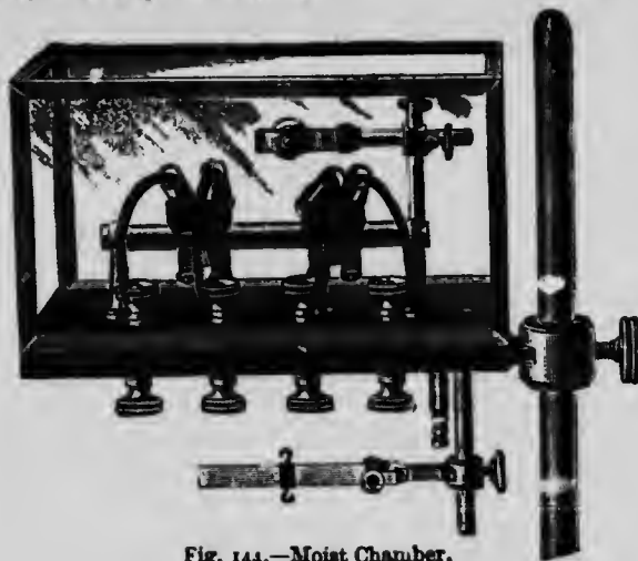
Fig. 144.—Moist Chamber.
