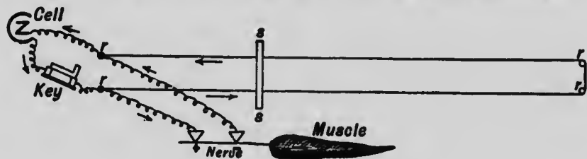
Fig. 186.—Simple rheochord.
