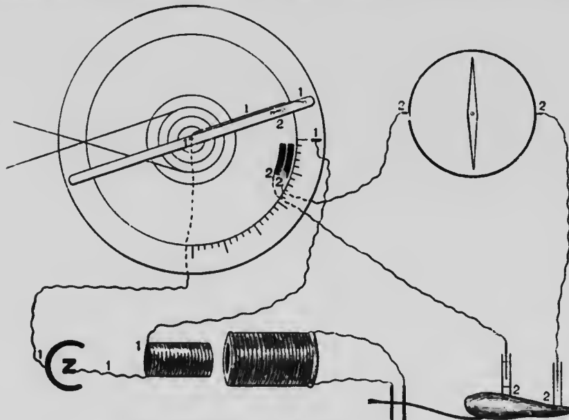
Fig. 109.—Scheme of a Rheotome. (Waller.)
