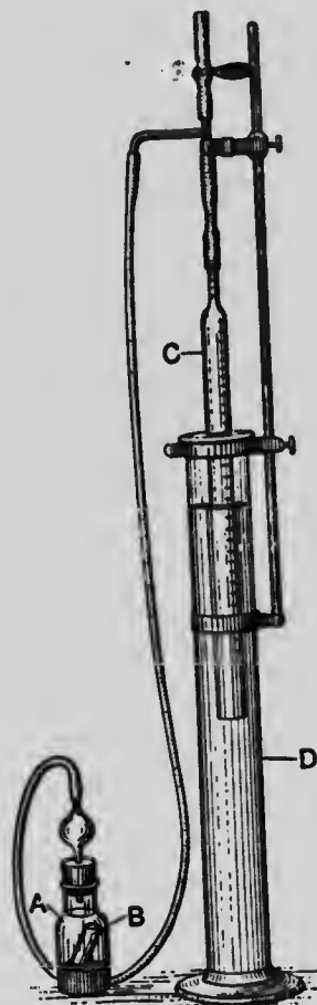
Fig. 432.—Dupré's urea apparatus.
