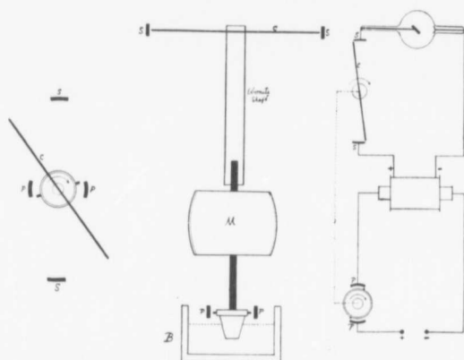
Fig. 32. Scheme of "Morton" Apparatus.
