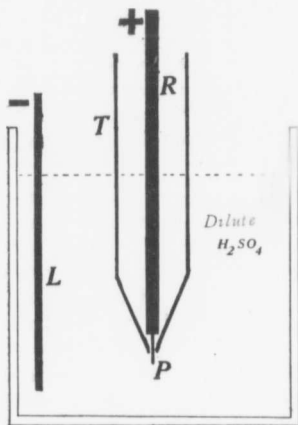
Fig. 35 Wehnelt Interrupter.
