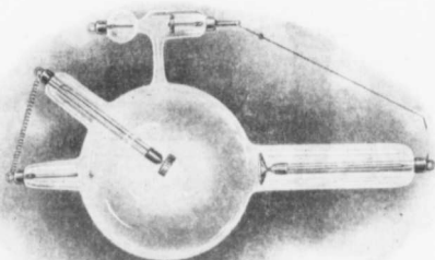
Fig. 18. Light Anode Muller Tube.
