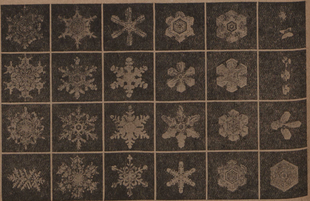
Vus au microscope, les cristaux de neige présentent les formes les plus variées et les plus élégantes, mais sont tous bâtis sur le type d'un polygone régulier à 6 côtés.
